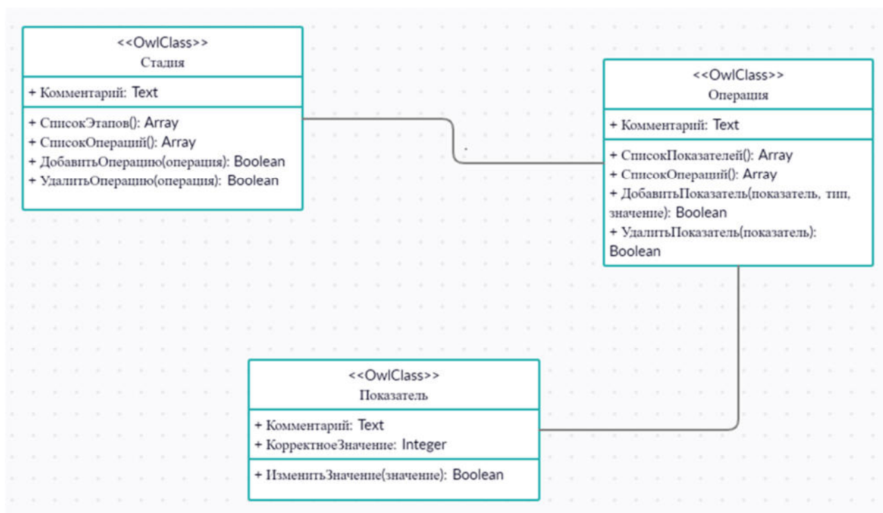
Рисунок 31 – Диаграмма классов онтологии описания процесса производства РФЛП
