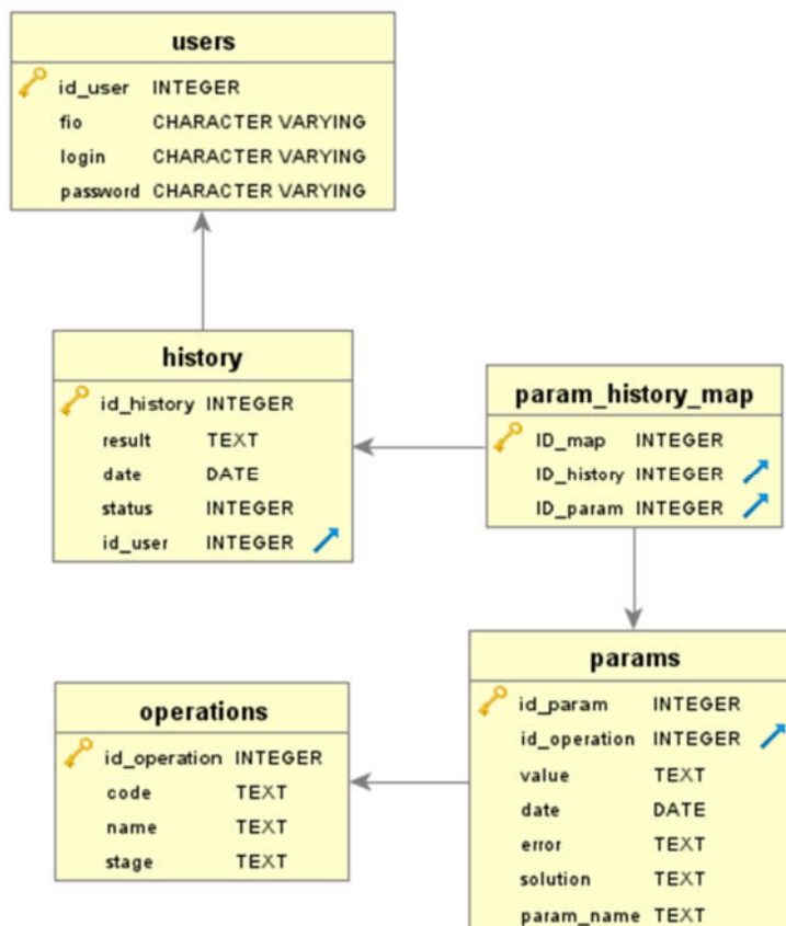
Рисунок 38 – Физическая модель базы прецедентов
