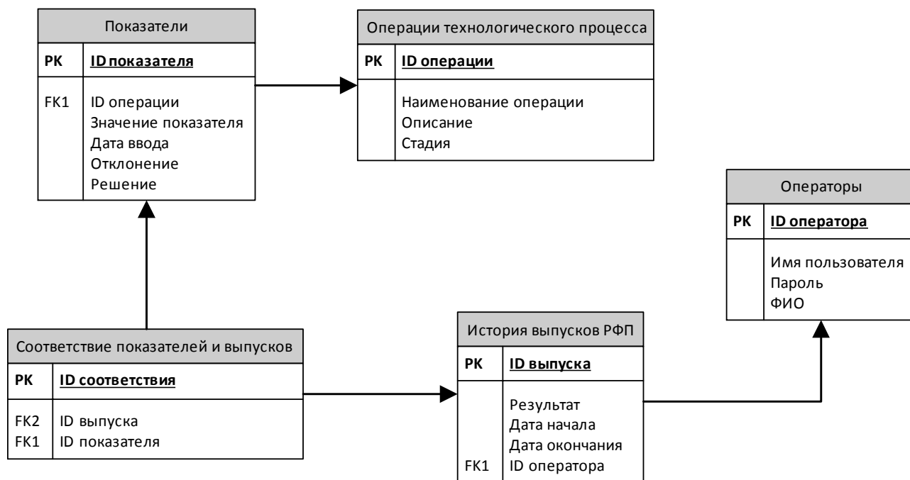
Рисунок 37 – Логическая модель базы прецедентов
