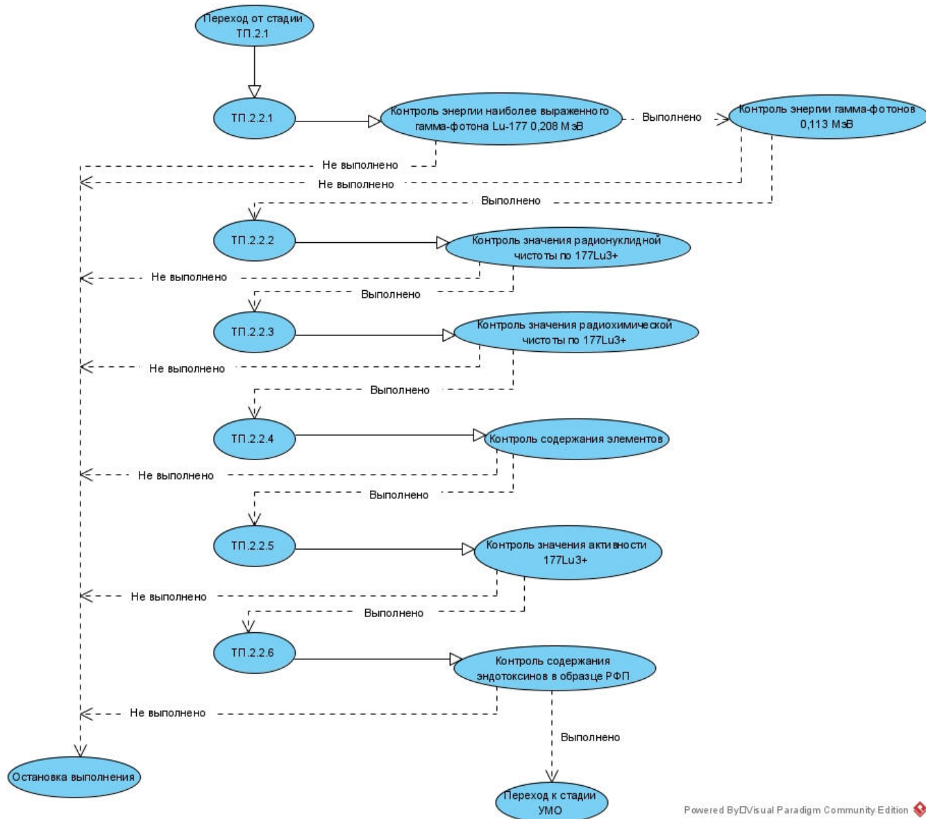
Рисунок 41 – Дерево переходов операций на стадии контроля качества РФЛП
