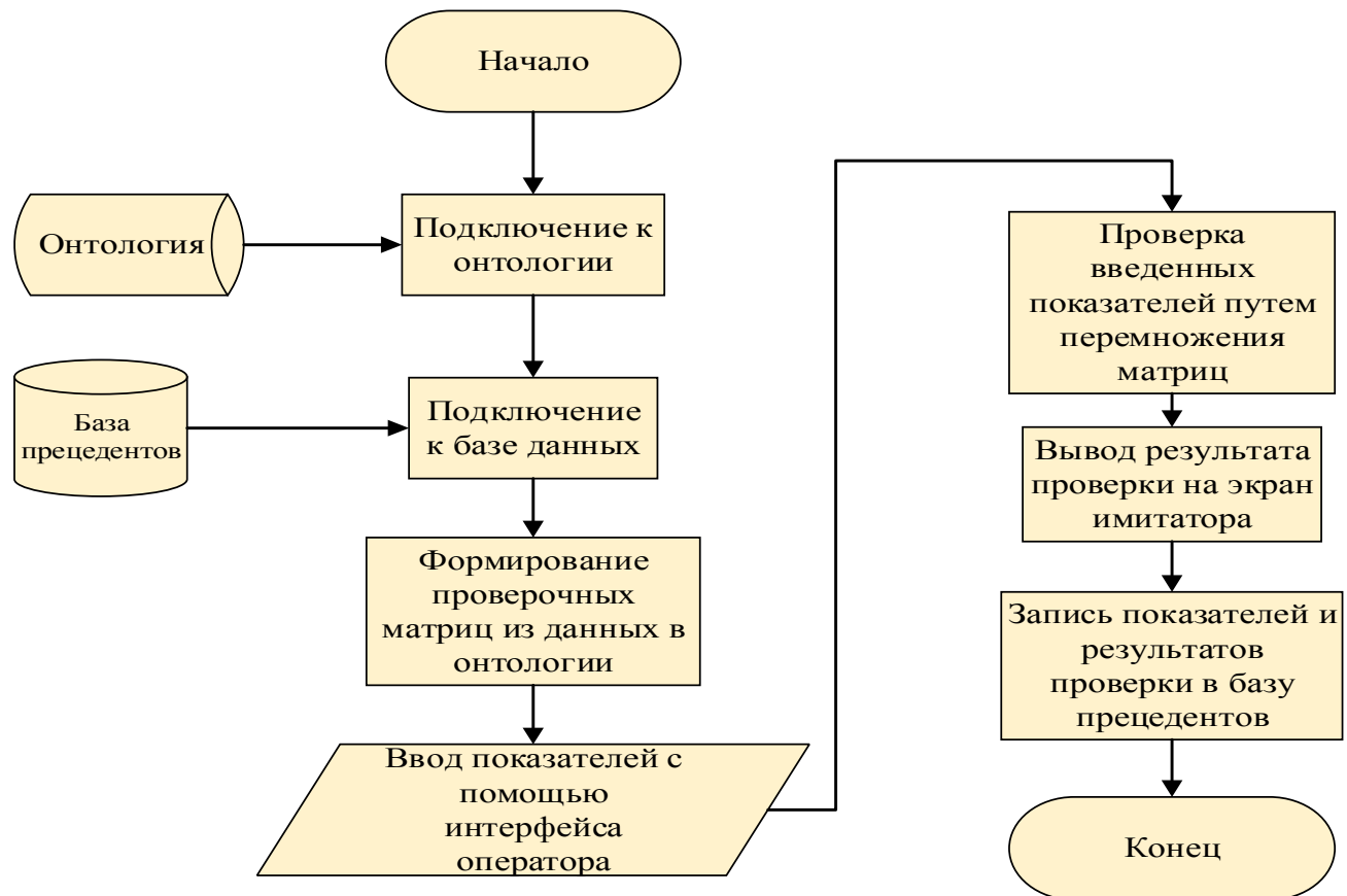
Рисунок 36 – Алгоритм работы имитатора
