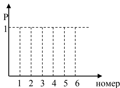
Рисунок 26 – Начальное распределение вероятностей
