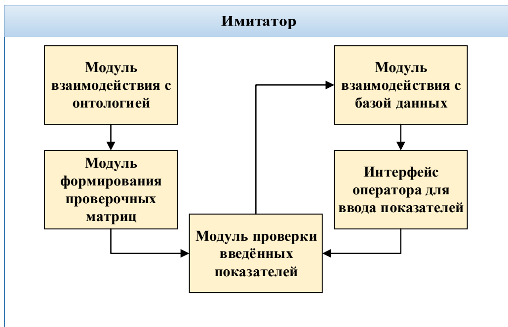
Рисунок 35 – Модульная схема имитатора ТП
