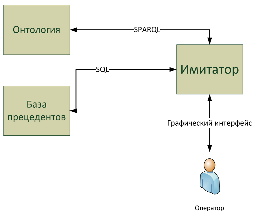
Рисунок 34 – Схема работы средства проверки выполнения этапов производства РФЛП
