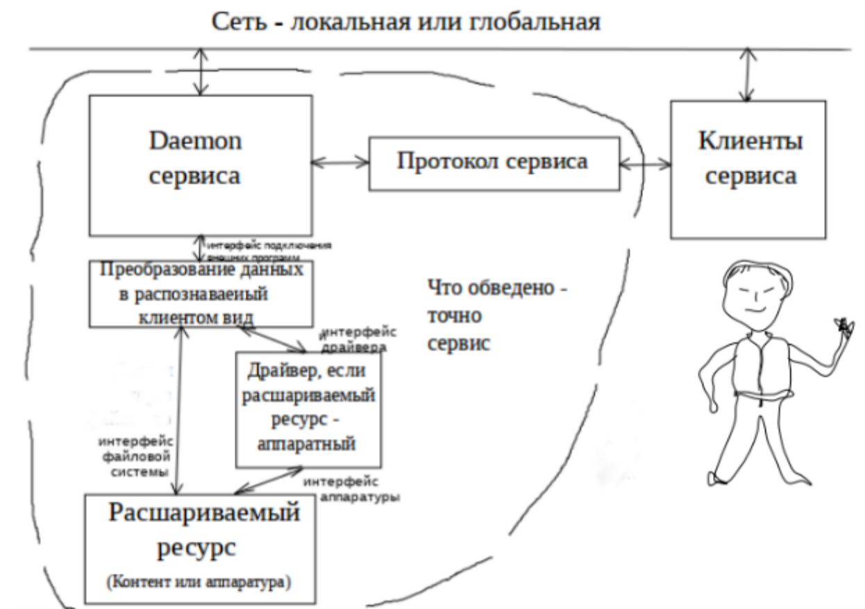
Рис. 39. Структура сетевого сервиса
