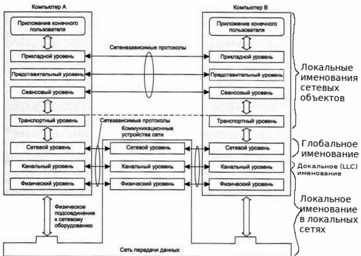
Рис. 10. Именование сетевых объектов на уровнях ЭМВОС
