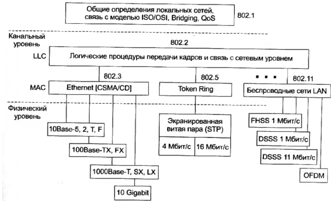
Рис. 7. Структура сетевых технологий. В каждой сетевой технологии показаны далеко не все релизы
