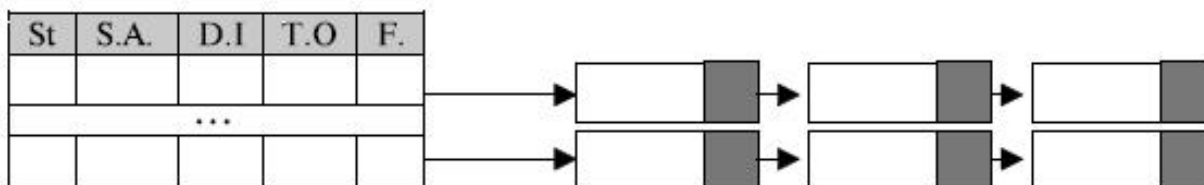
Рис. 27. Таблица реасSEMBЛИРОВАНИЯ
