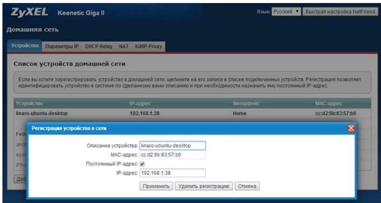
Рис. 2. Назначение ip-адреса
