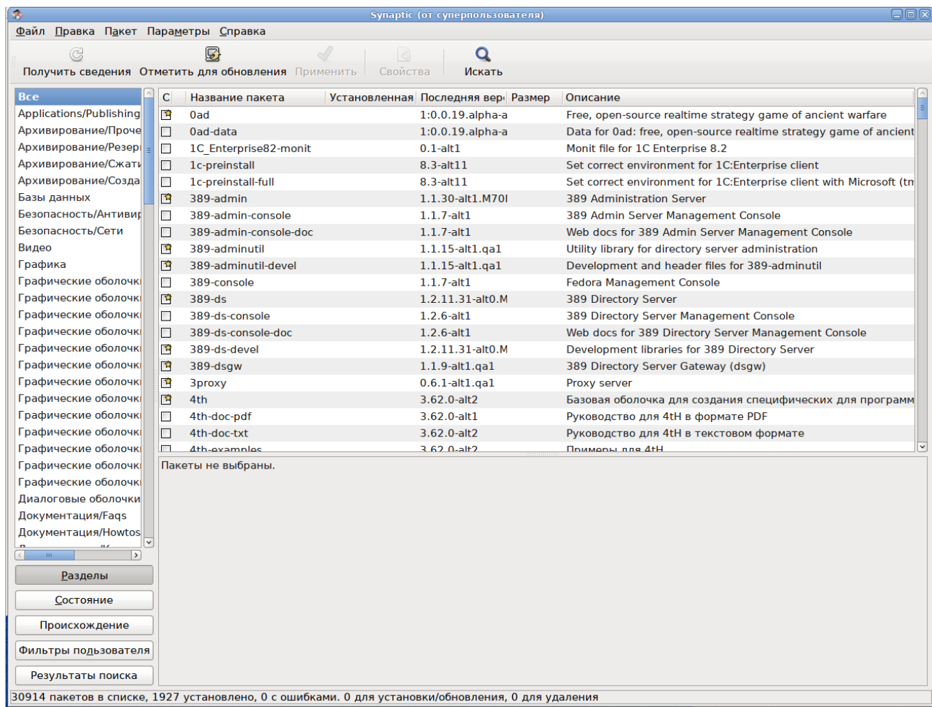
Рис. 2. Окно synaptic
