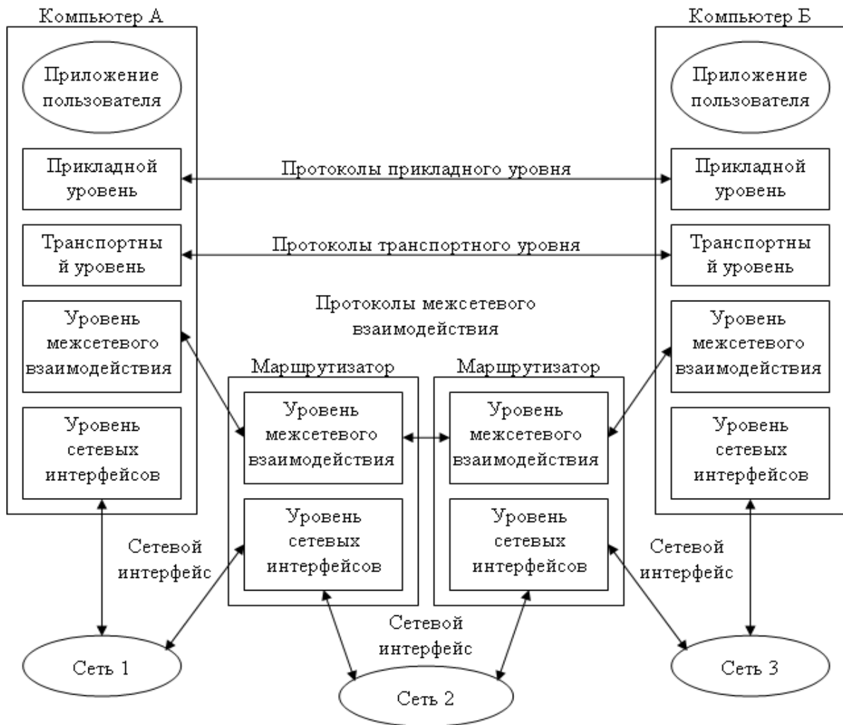
Рис. 18. Сетезависимые и сетезависимые уровни стека TCP/IP. Широкие серые стрелки определяют логические взаимодействия (логическую топологию). Чёрные тонкие стрелки — физические взаимодействия (физическую топологию)
