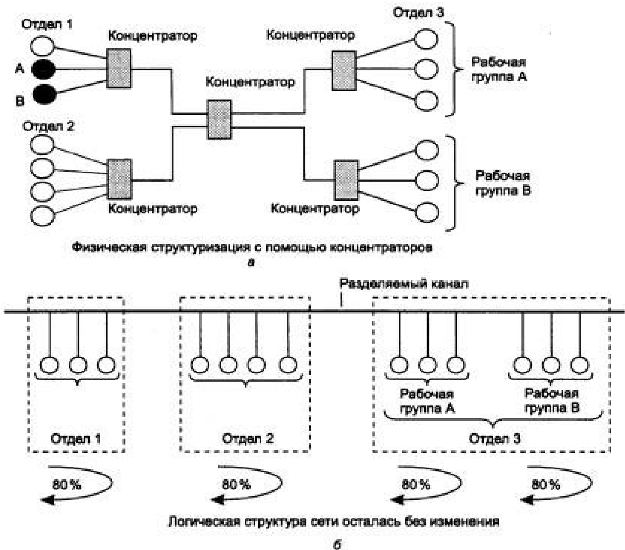
Рис. 9. Физическая и логическая структура сети — две большие разницы. 80% трафика в каждом сегменте являются локальными, но концентраторы транслируют трафик на все компьютеры. То есть, в сети с концентраторами каждый компьютер «слышит» любой другой компьютер, подключенный к разделяемому каналу
