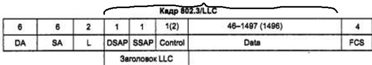
Рис. 8. Кадр MAC. В середине фигурной скобкой выделен инкапсулированный кадр LLC
